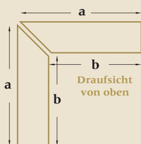
Verkröpfungsschnitt für Hausecken Länge inkl. Schnitt = a , Länge zzgl. Schnitt = b
